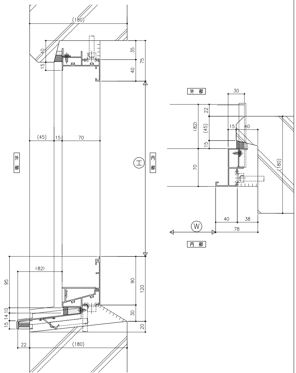
アゴ付納まり S:1/6
